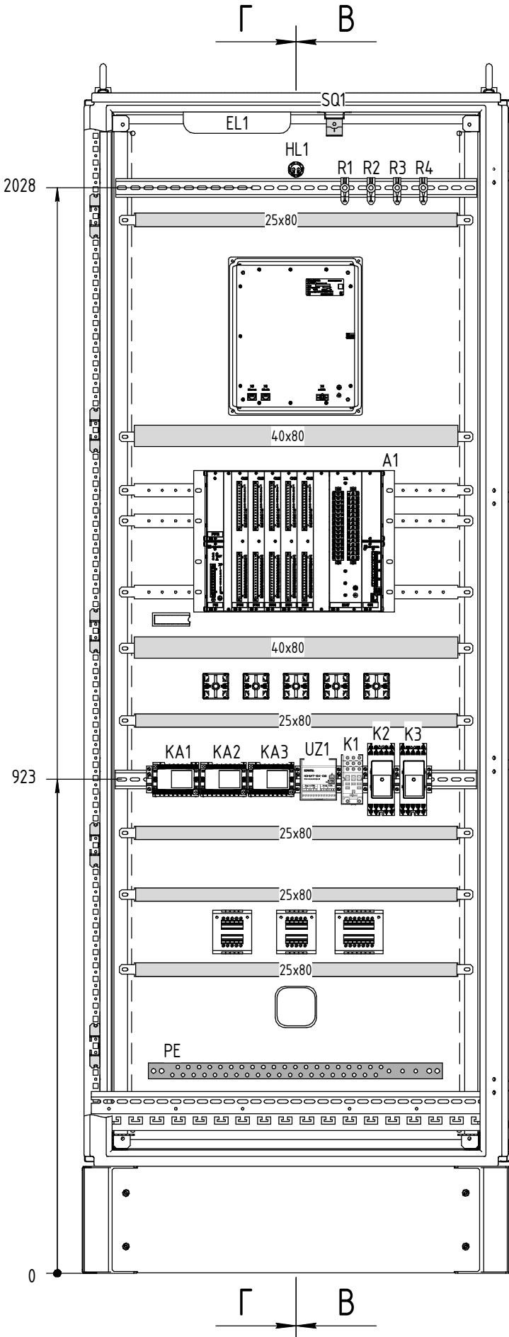
Вид сзади Дверь, ряды зажимов и вертикальные короба условно не показаны
