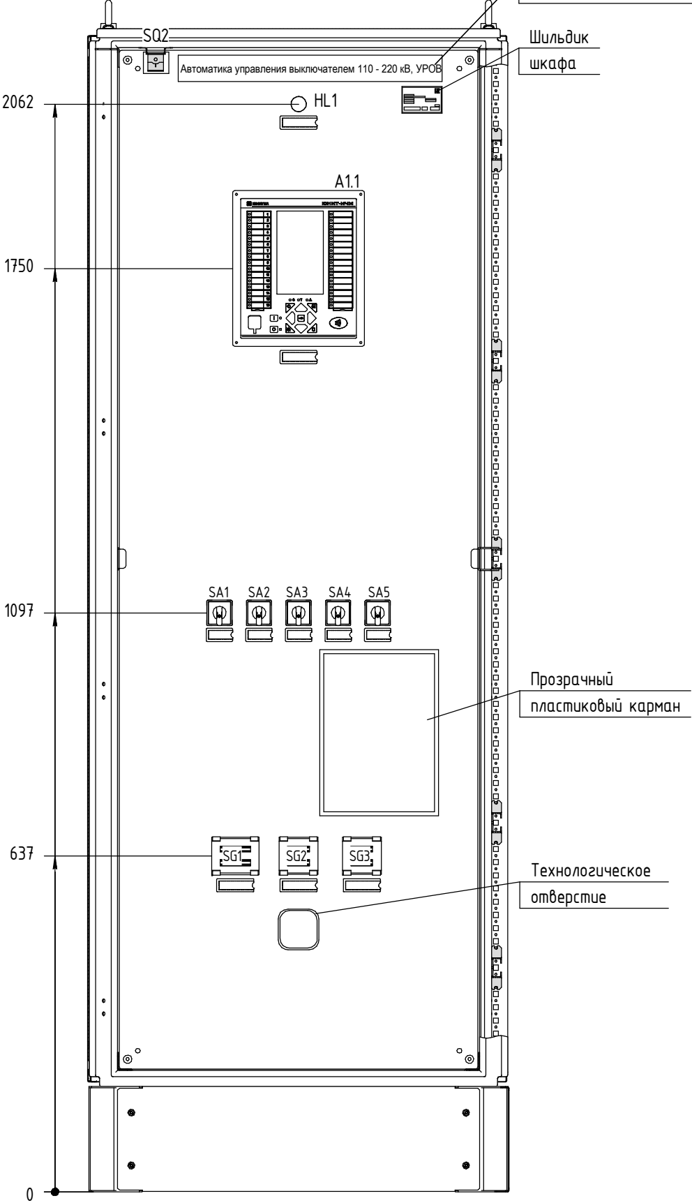
Вид спереди Дверь условно не показана
